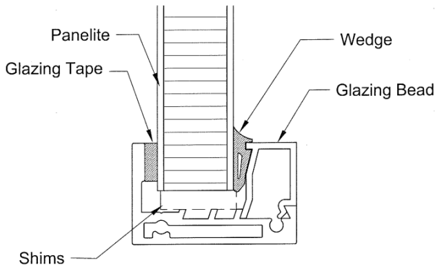
Pre-Fab Flush Edge
